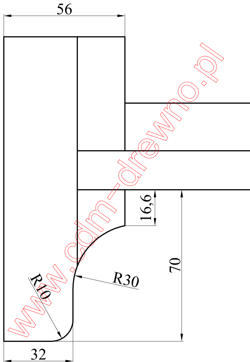
detal A
